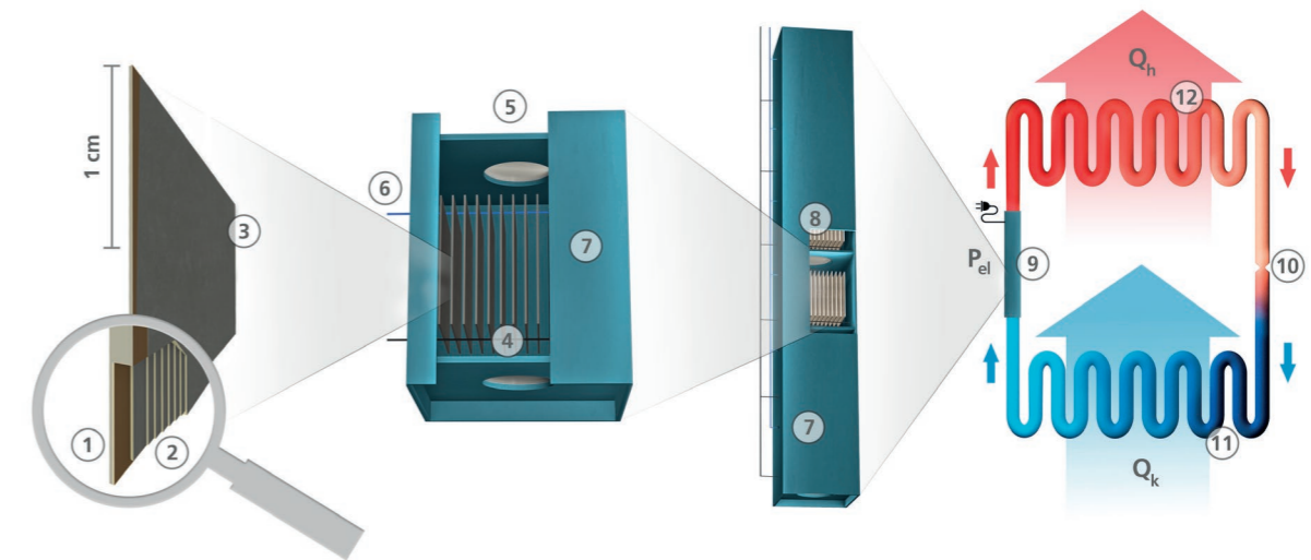
Aufbau einer elektrokalorischen (EK) Wärmepumpe: Die EK-Komponenten bestehen aus den EK-Materialien (1) inklusive Elektroden (2) und Beschichtung (3). Mehrere dieser Komponenten (4) sowie Rückschlagventile (5) und elektrische Zuleitung (6) werden in ein gasdichtes Gehäuse (7) integriert und zu einem EK-Segment zusammengefügt. Mehrere solcher EK-Segmente (8) in Reihe geschaltet ergeben das EK-System (9) und zusammen mit einer Drossel (10), dem Verdampfer (11) und dem Kondensator (12) eine EK-Wärmepumpe.
